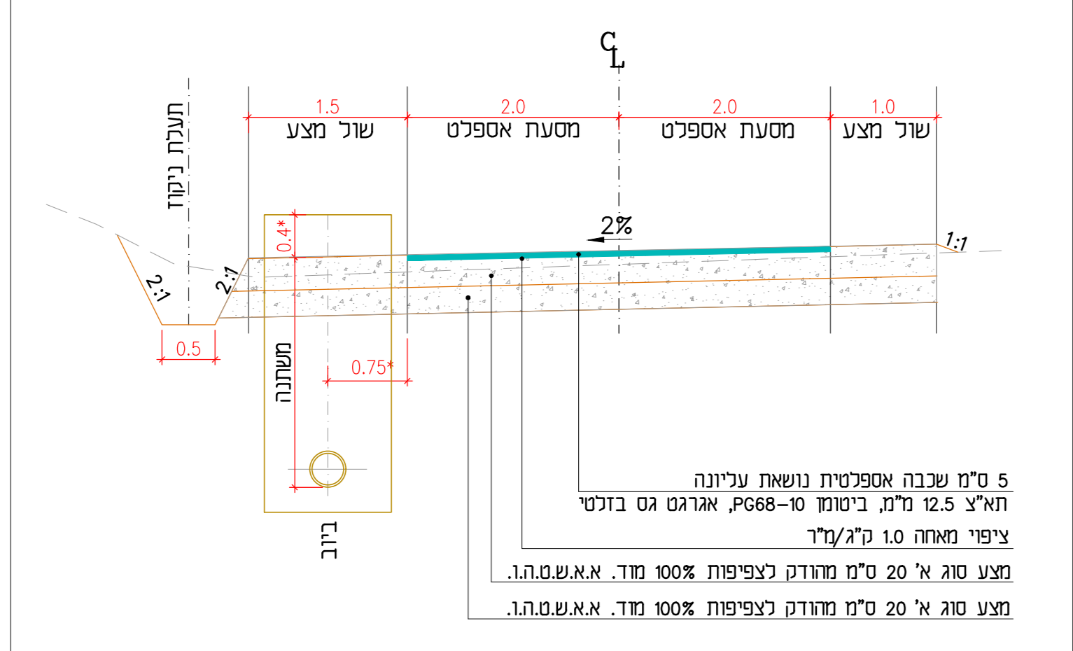
דרר שרות מאספלט חתך טיפוסי לכביש ברוחב 4 מ'
